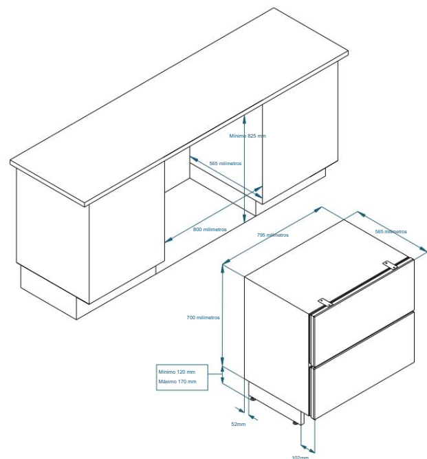
Cajón frigorífico para montaje de frente de mueble. Medidas recomendadas para los frentes de mueble a colocar:
