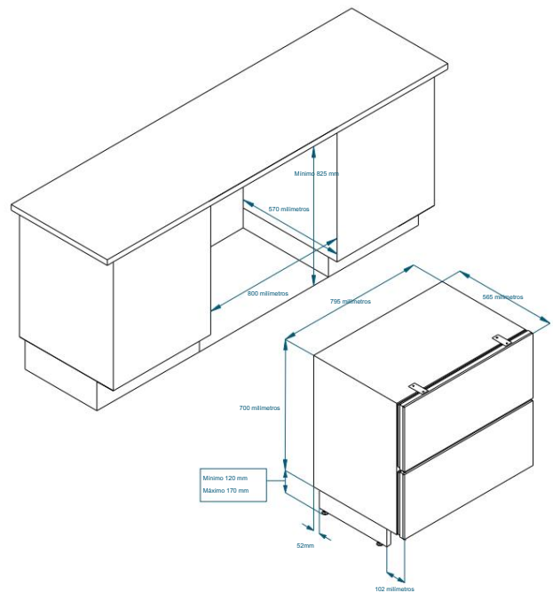
Cajón congelador para colocar frente de mueble. Medidas recomendadas de los frentes de muebles a instalar: Ancho: 795 mm / Alto: 341-348 mm
